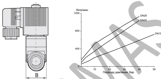
Диаграмма 1. Зависимость расхода от давления
