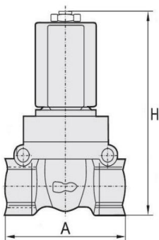
Рисунок 1. Эскиз
