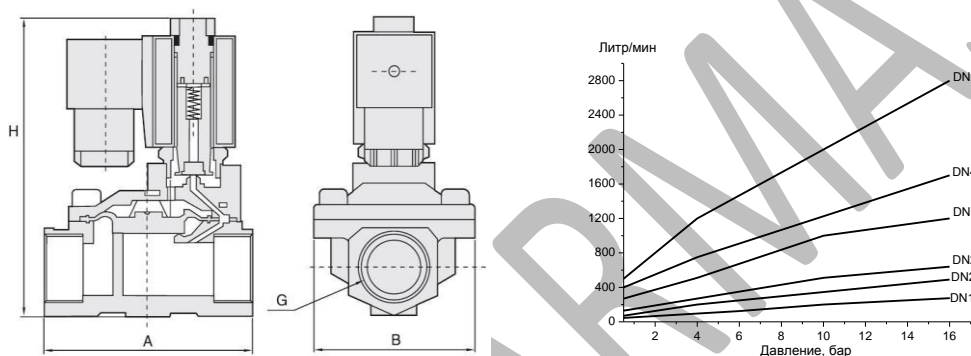
Рисунок 1. Эскиз
